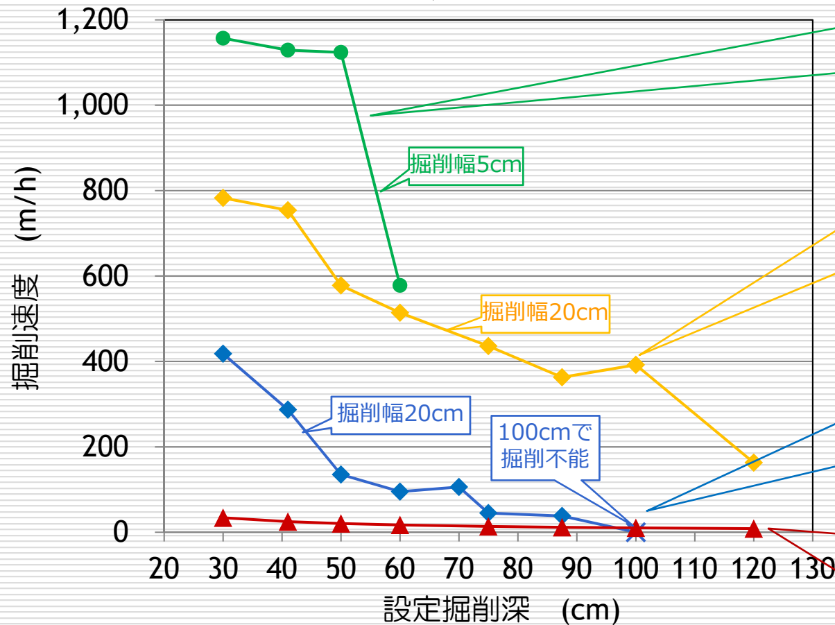
▼設定掘削深と掘削速度の関係
