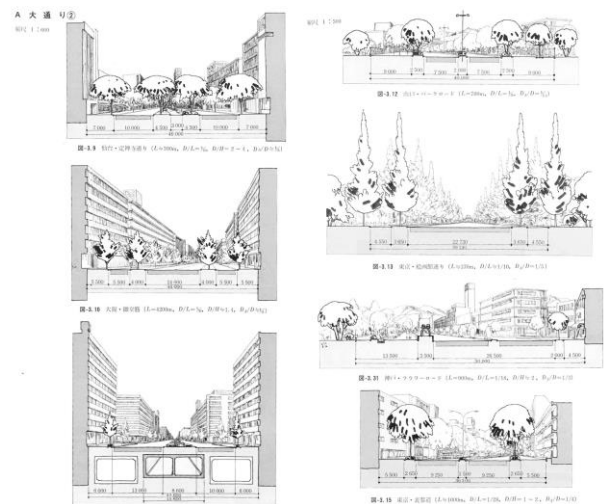
図-2 街路のプロポーショナルの実例(参考文献 9) pp36-37より引用)
