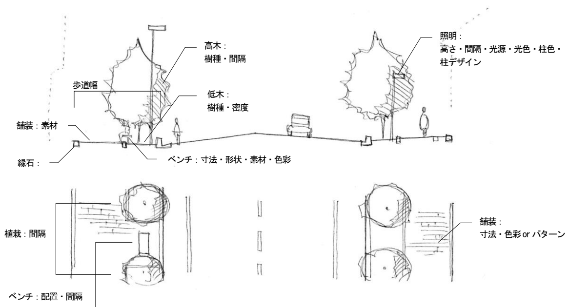
図-1 一般的な道路の横断面図および平面図
