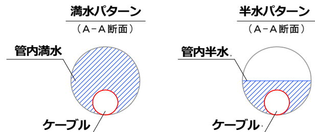
図-11 滞留水の再現パターン
