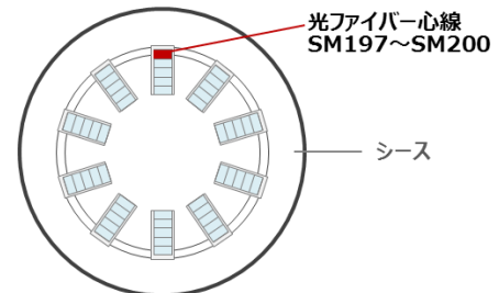
図-12 光ケーブル断面イメージと測定箇所
