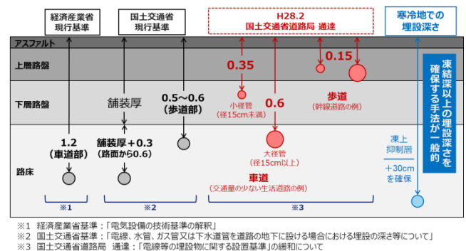
図-2 我が国の埋設深さと寒冷地での埋設深さの比較(黒:現在, 赤:H28.2月の通達, 青:寒冷地)
