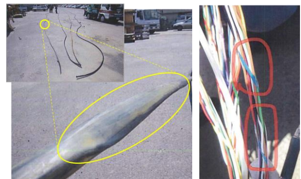
写真-6 通信用メタルケーブルの凍結圧迫・断線事例 (左:外装の変形 右:内部ケーブルの接続障害)
