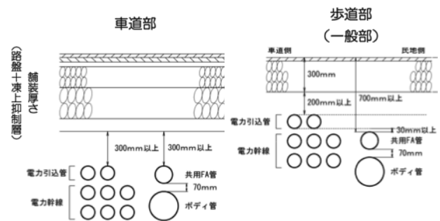
図-8 北海道における電線共同溝の埋設深さ基準 左)車道部、右)歩道部 (電線共同溝技術マニュアル 9) より引用・加筆)
