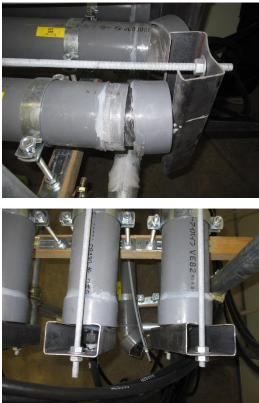
写真-8 凍結後の供試体蓋部 (上:満水 下:半水)
