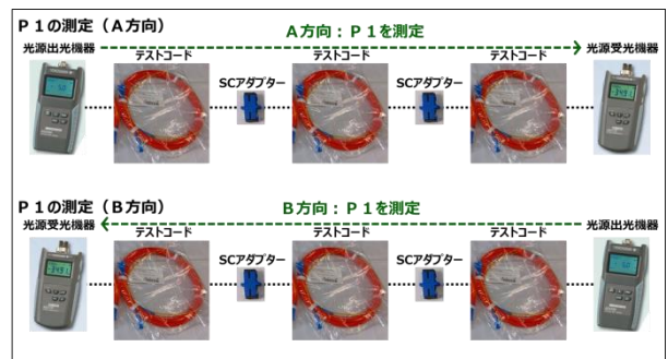
図-13 基準値 P1 の測定方法
