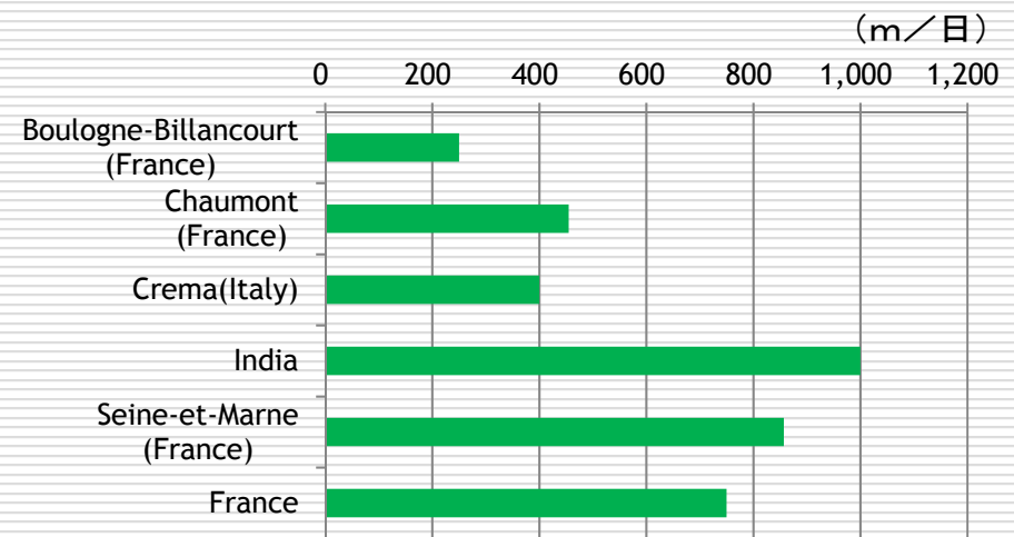
トレンチャーによる日当たり掘削延長
