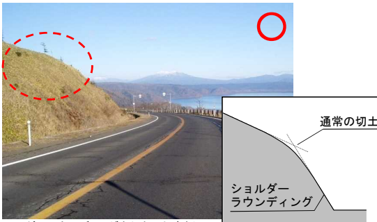
ショルダーラウンディングを行なった事例 のり肩を丸めることで、人工的な印象が緩和される。
