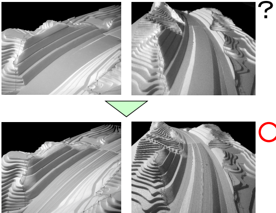
切土面が連続している場合には、地山との関係性を考慮した谷を造成することによって切土面の違和感を解消することを検討する。
