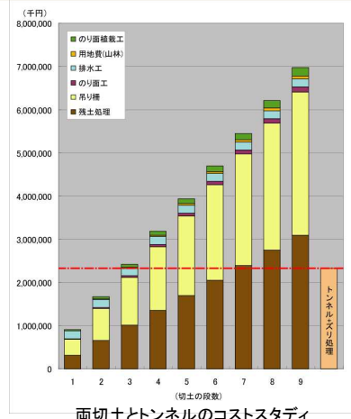
両切土とトンネルのコストスタディ
