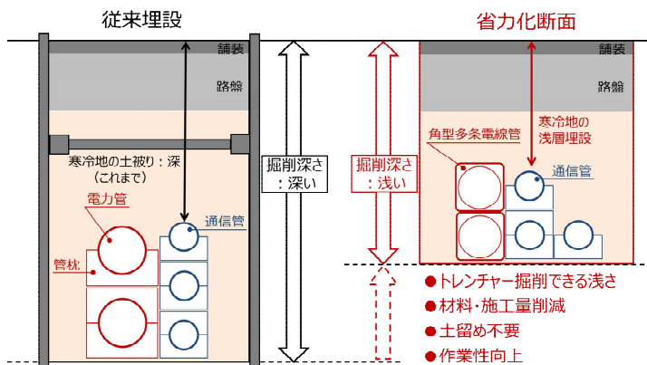
▲省力化断面のイメージ
