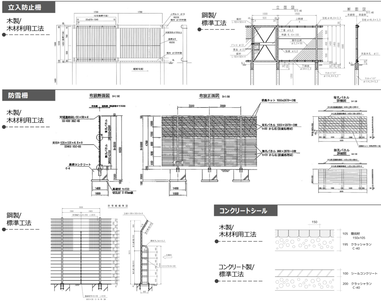
図-2 木材利用にかかる効果の算定に用いた構造物の概略図
