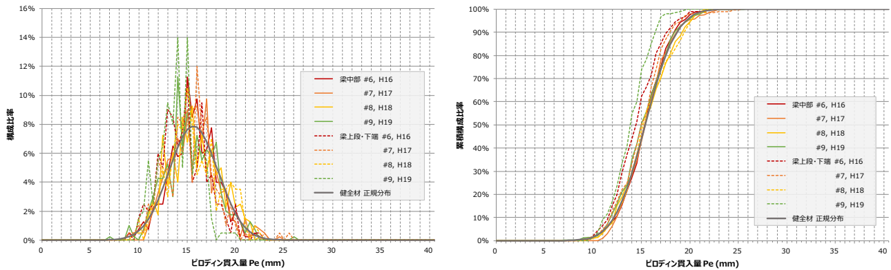
図-9 健全部材のピロディン貫入量分布とそれらから算出した平均値・標準偏差に基づく正規分布モデル
