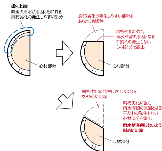
図-19 腐朽劣化の進行を抑制する横架材構造の試案
