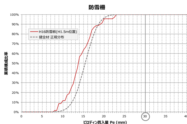
図-10 防雪柵防雪板に関するピロディン計測値の分布
